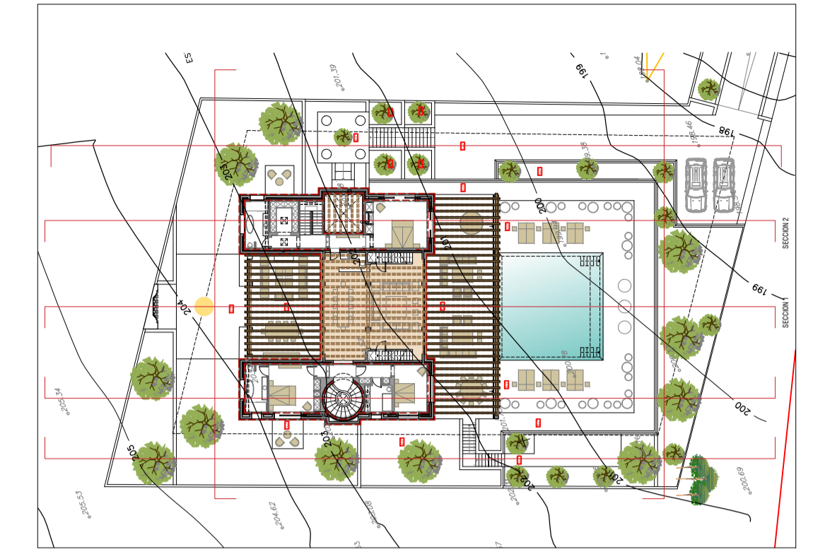
PLANTA PRIMERA 1/500
