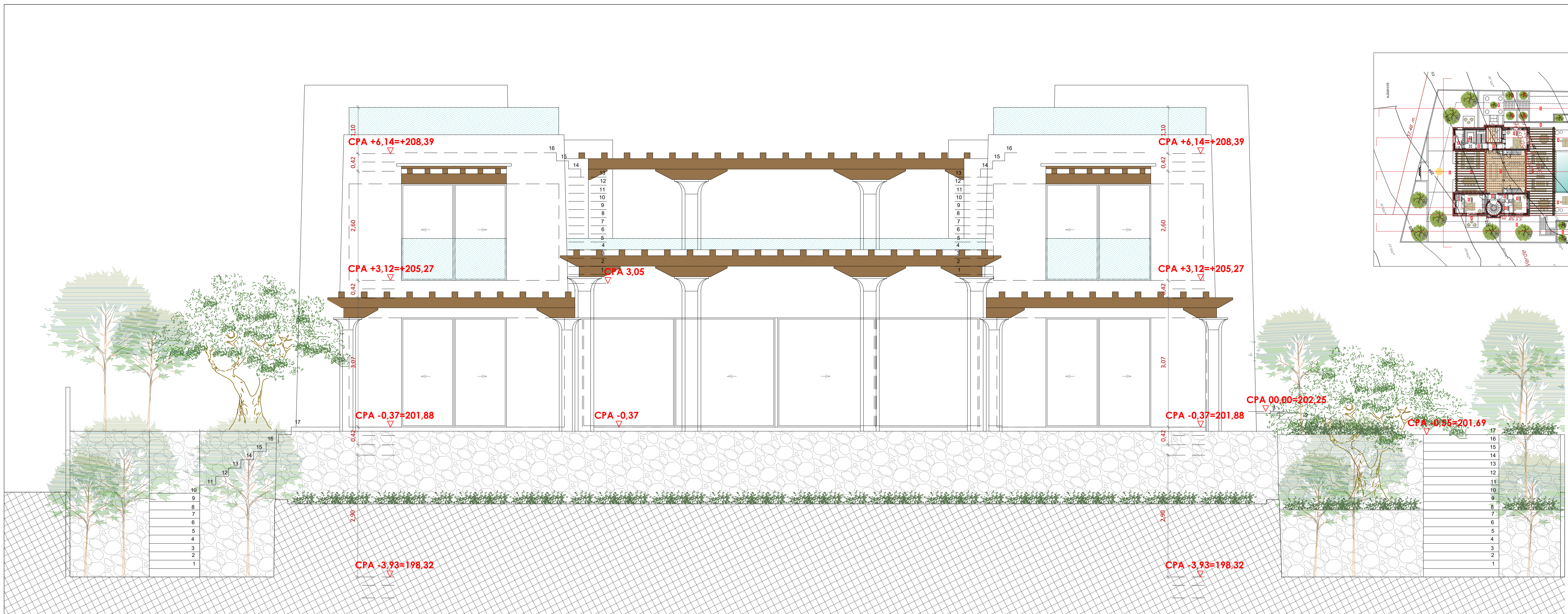
ALZADO SUR
